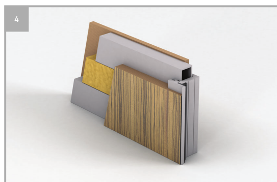
Montáž na MDF panely
