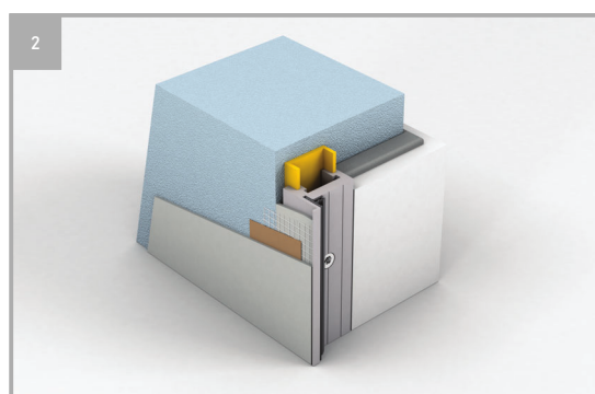
Montáž na siporex/porobeton
