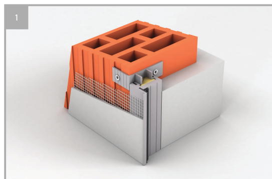
Montáž na cihlovou zeď
